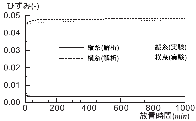
図 22. 初期張力 6.7kgf/cm の 2 軸クリープ解析
