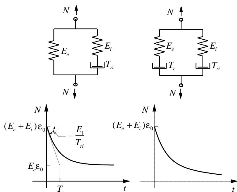
(a) 3要素 Maxwell モデル (b) 4要素 Maxwell モデル
