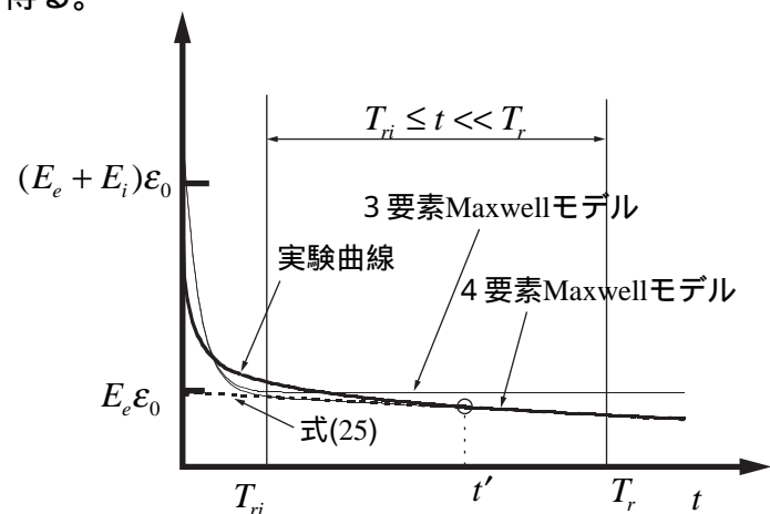
図 11. T_r の推定 ( 方向 )
