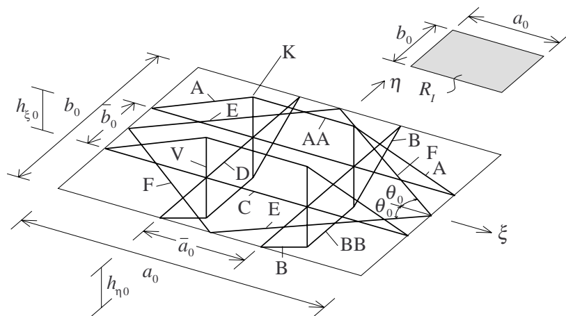
図1. 織構造格子モデル
