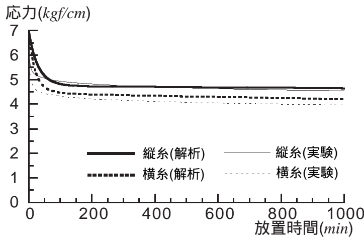
図 17. 初期張力 7.0kgf/cm の等 2 軸初期応力緩和解析
