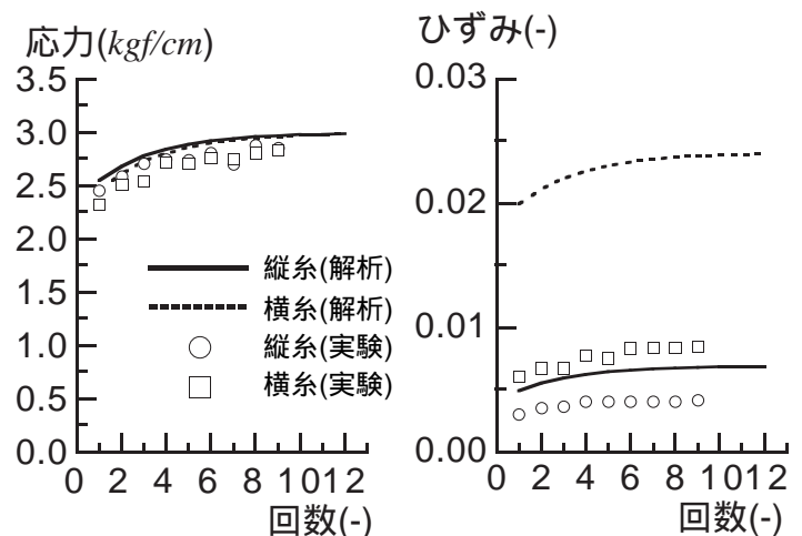
図 27. 繰り返し载荷による 2 軸応力緩和解析 (初期張力 3.0kgf/cm)
