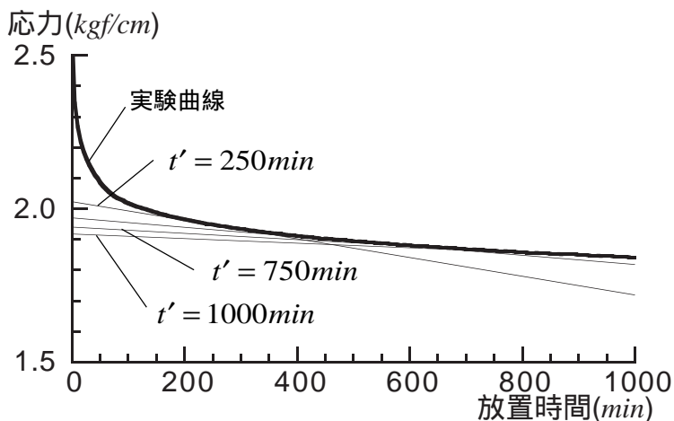
図 10. E_e \epsilon_0 の推定 ( 方向 )
