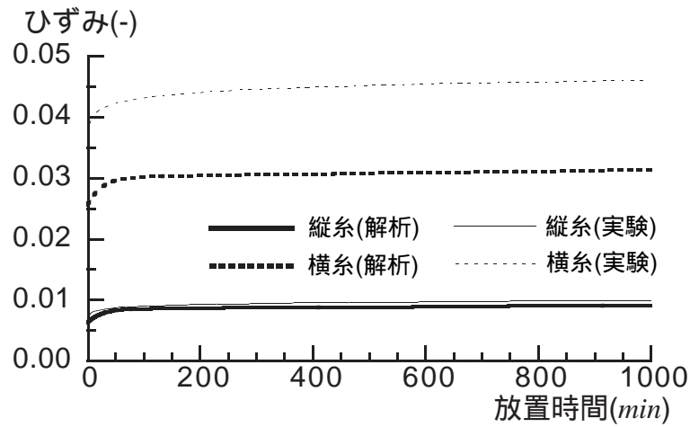
図 19. 初期張力 3.3kgf/cm の 1 軸クリープ解析
