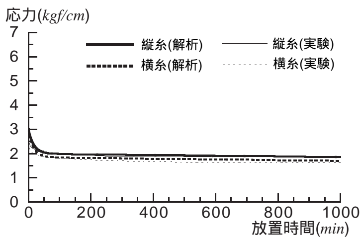
図 15. 初期張力 3.0kgf/cm の等 2 軸初期応力緩和解析
