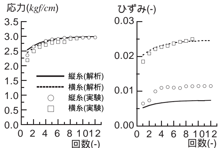
図 26. 繰り返し载荷による 1 軸応力緩和解析 (初期張力 3.0kgf/cm)
