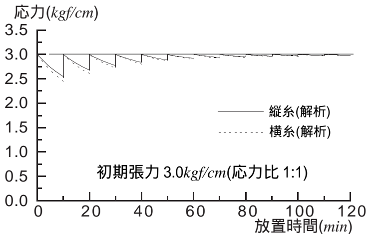
図 24. 繰り返し载荷を受ける応力緩和解析の様子 (応力 時間関係)
