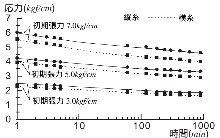
図 7. 2 軸応力緩和試験の結果
