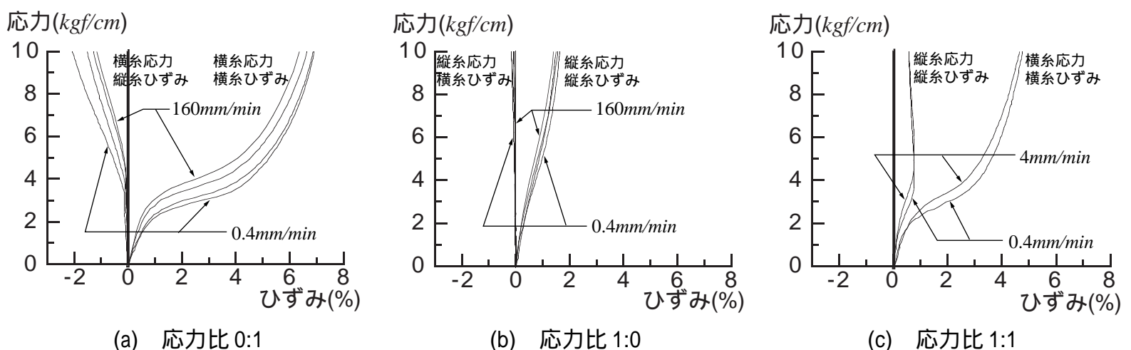
図 4. 引張速度を変化させることによる応力・ひずみ関係への影響
