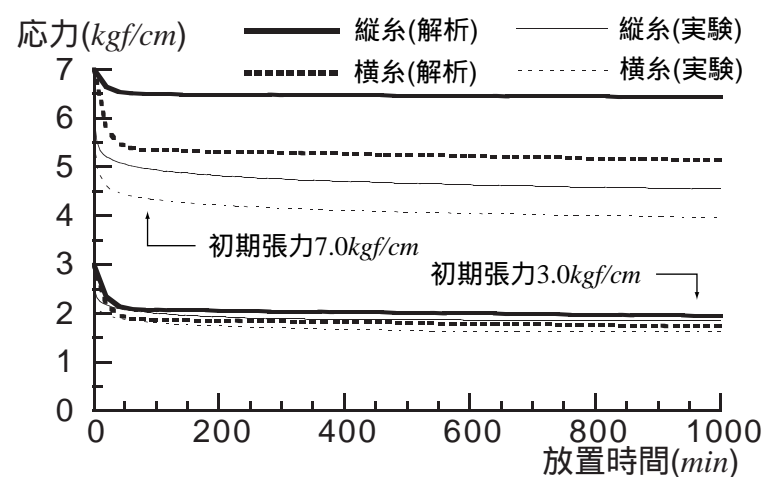
図13. 表5の値を用いた2軸応力緩和解析
