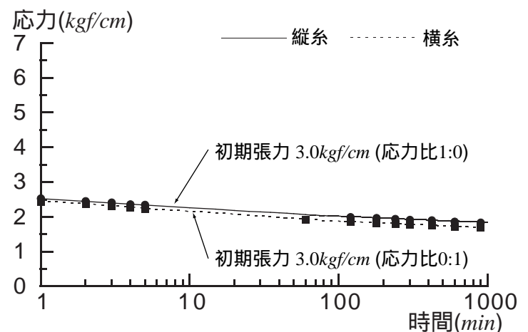
図 8. 1 軸応力緩和試験の結果
