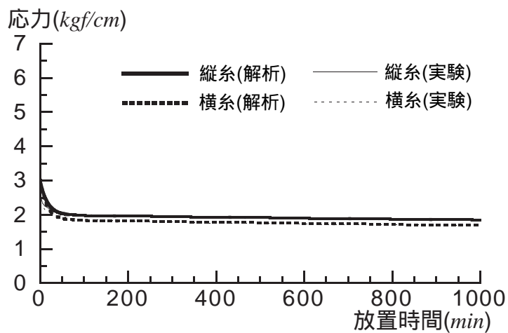
図 14. 初期張力 3.0kgf/cm の 1 軸応力緩和解析
