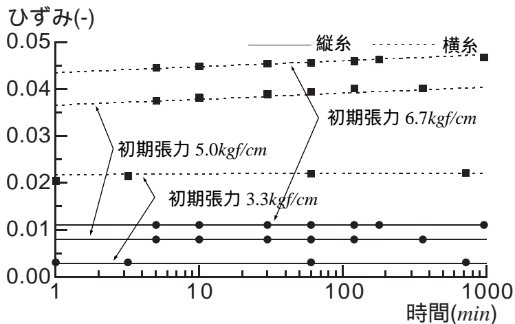
図 5. 2 軸クリープ試験の結果
