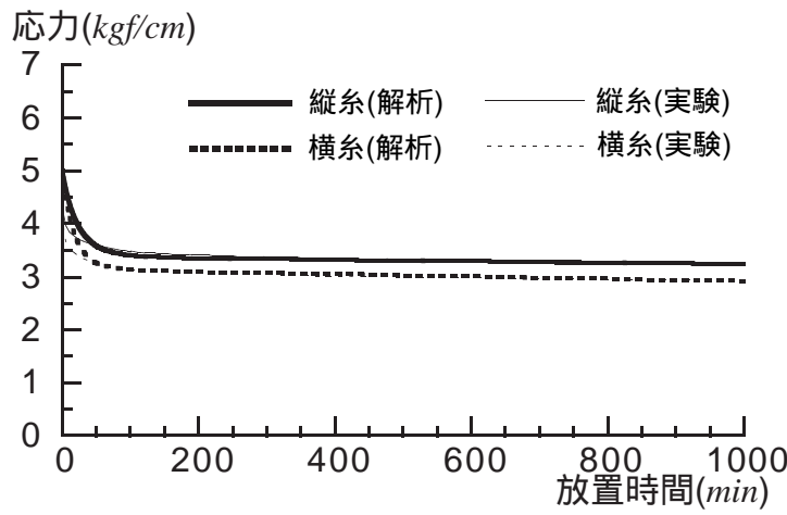
図 16. 初期張力 5.0kgf/cm の等 2 軸初期応力緩和解析
