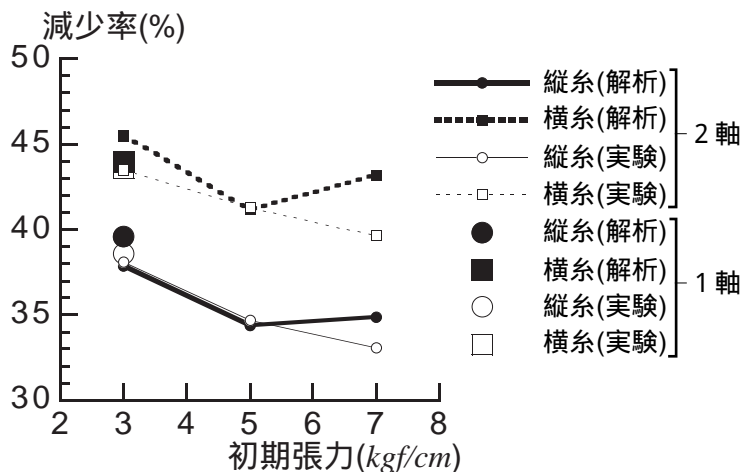
図18. 緩和応力の減少率
