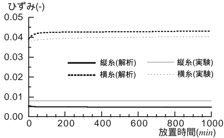
図 21. 初期張力 5.0kgf/cm の 2 軸クリープ解析
