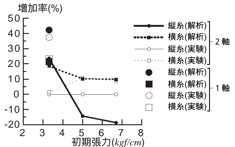
図23. クリープひずみの増加率
