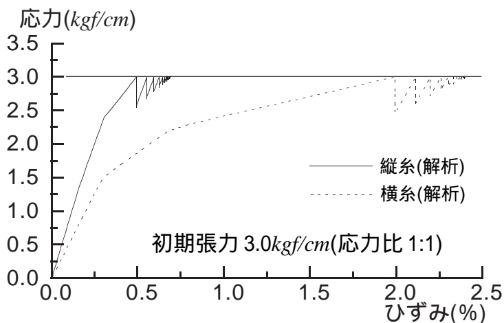
図 25. 繰り返し载荷を受ける応力緩和解析の様子 (応力 ひずみ関係)
