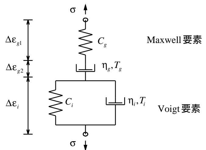
図2. 4要素Voigtモデル
