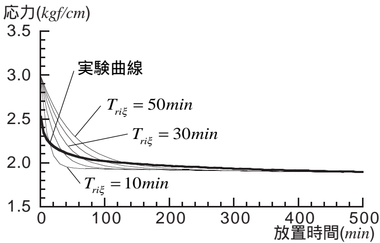
図12. T_{ri} の推定 (方向)
