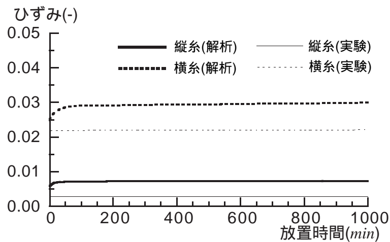
図 20. 初期張力 3.3kgf/cm の 2 軸クリープ解析
