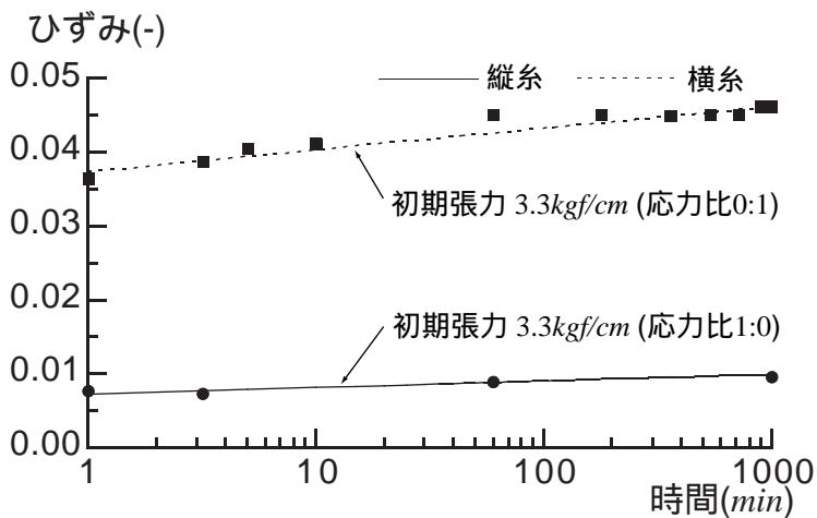
図 6. 1 軸クリープ試験の結果
